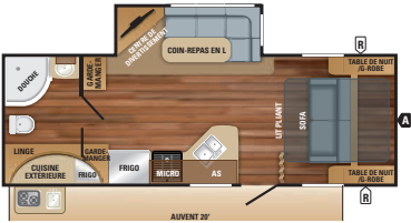
WHITE HAWK | 23MRB OPTION A Longueur ext. : 28' 2" Hauteur ext. : 131" Poids à vide (lbs) : 5 560 Personnes : 2-4
