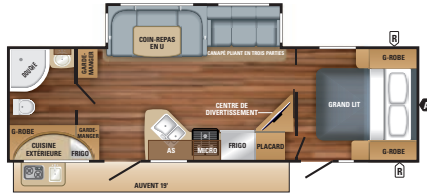
WHITE HAWK | 27RB OPTIONS : A, B Longueur ext. : 32' 8" Hauteur ext. : 134" Poids à vide (lbs) : 6 500 Personnes : 2-6
