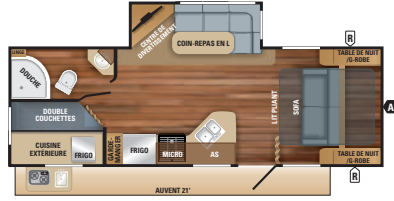
WHITE HAWK | 24MBH OPTION A Longueur ext. : 29' 2" Hauteur ext. : 131" Poids à vide (lbs) : 5 680 Personnes : 6-8
