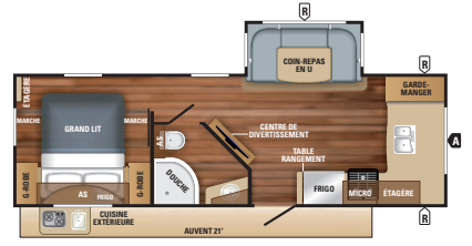
WHITE HAWK | 25FK OPTION A Longueur ext. : 30' 2" Hauteur ext. : 132" Poids à vide (lbs) : 5 750 Personnes : 2-4
