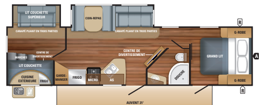
WHITE HAWK | 31BH OPTIONS : A, B Longueur ext. : 37' 6" Hauteur ext. : 135" Poids à vide (lbs) : 7 775 Personnes : 4-8
