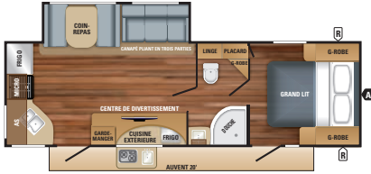
WHITE HAWK | 26RK OPTIONS : A, B Longueur ext. : 28' 9" Hauteur ext. : 131" Poids à vide (lbs) : 6 055 Personnes : 2-6
