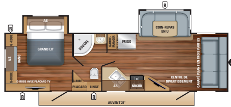
WHITE HAWK | 29FLS OPTION A Longueur ext. : 34' 5" Hauteur ext. : 134" Poids à vide (lbs) : 6 635 Personnes : 4-6
