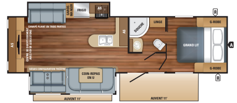
WHITE HAWK | 29RE OPTION A Longueur ext. : 35' 0" Hauteur ext. : 136" Poids à vide (lbs) : 7 195 Personnes : 4-6
