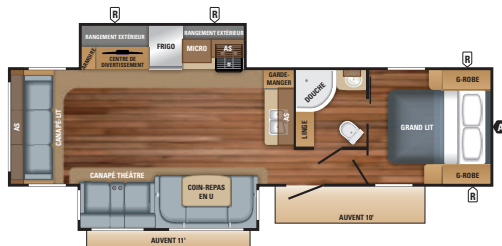
WHITE HAWK | 31RL OPTION A Longueur ext. : 36' 11" Hauteur ext. : 136" Poids à vide (lbs) : 7 560 Personnes : 4-6
